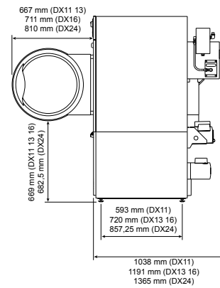
Вид с боку DX 11
