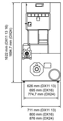
Вид сзади DX 11
