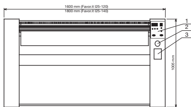
ВИД СПЕРЕДИ FAVOR.IT | 25-120, FAVOR.IT | 25-140
