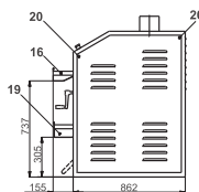
ВИД СБОКУ
