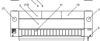
ВИД СЗАДИ – МОДЕЛЬ С ПАРОВЫМ НАГРЕВОМ
