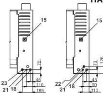
МОДЕЛЬ С ЭЛЕКТРИЧЕСКИМ НАГРЕВОМ
