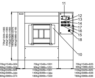
Вид БОКУ МВ 70 90 110 140 180
