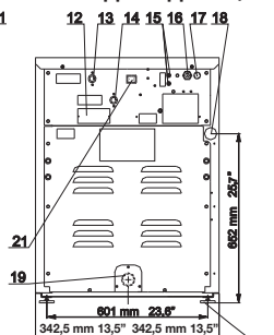
ВИД СЗАДИ Р6, Р7
