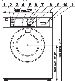
ВИД СПЕРЕДИ Р6, Р7
