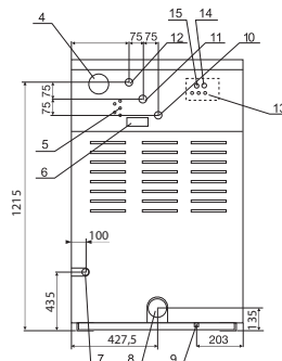
ВИД СЗАДИ RS 18 22
