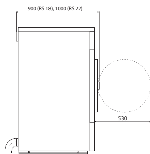
ВИД СБОКУ RS 18 22
