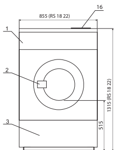
ВИД СПЕРЕДИ RS 18 22
