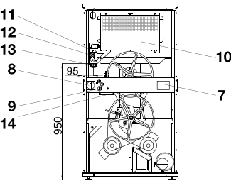
ВИД СЗАДИ Т 9 (МОДЕЛЬ С ГАЗОВЫМ НАГРЕВОМ)
