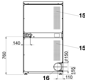
ВИД СЗАДИ Т 9 (МОДЕЛЬ С ЭЛЕКТРИЧЕСКИМ НАГРЕВОМ)
